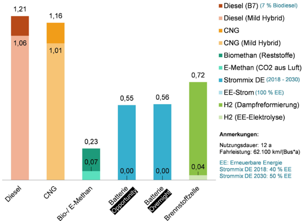
Abbildung 8: Well-to-Wheel-Emissionen des Linienbetriebs nach Antriebsart (ohne Batterie- und Fahrzeugherstellung)
