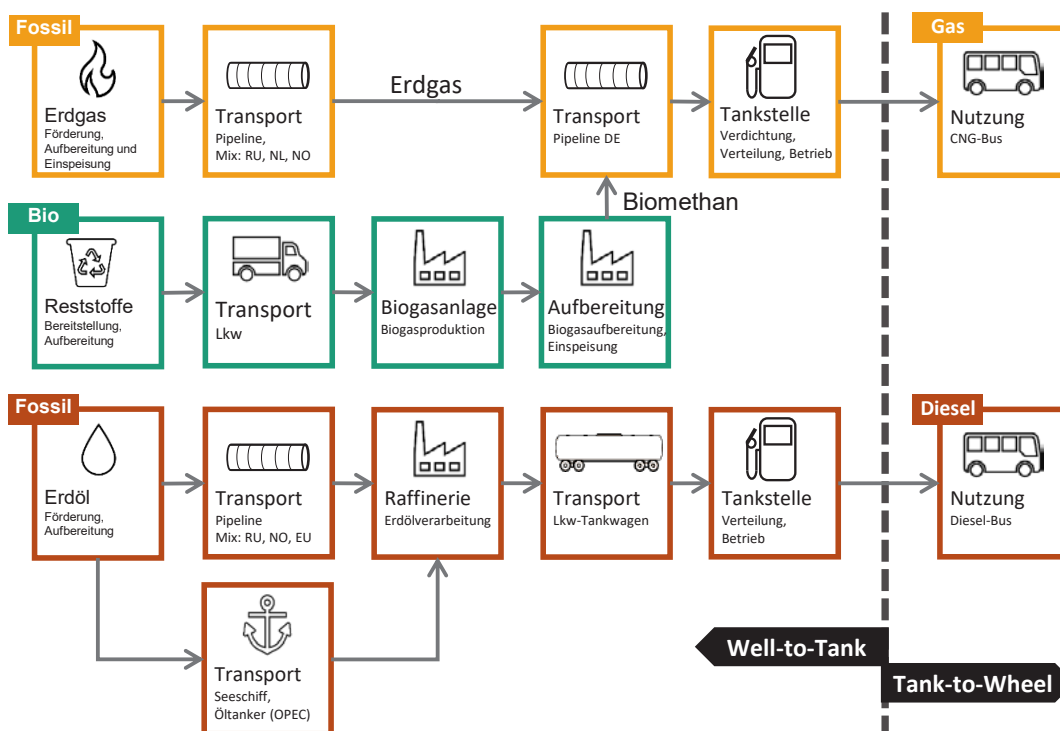
Abbildung 7: Bestandteile der Well-to-Wheel-Prozesskette bei Gas- und Dieselmotoren
