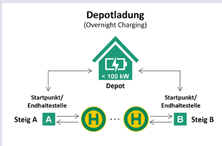
Abbildung 5: Schematische Darstellung des Ladekonzepts „Depotladung“
