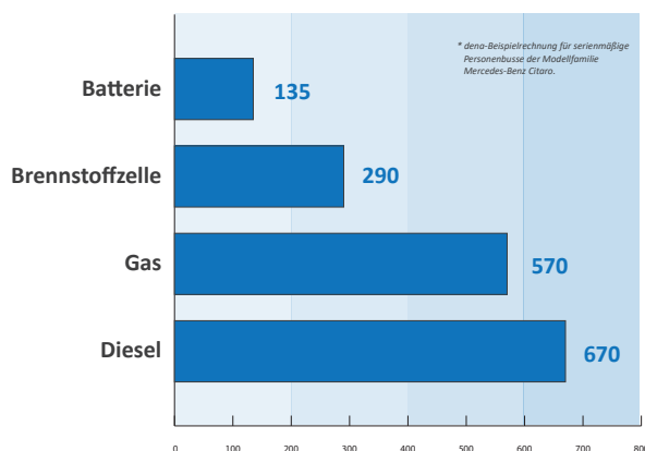
Abbildung 1: Reichweiten für Linienbusse nach Antriebsart 2 [6]
