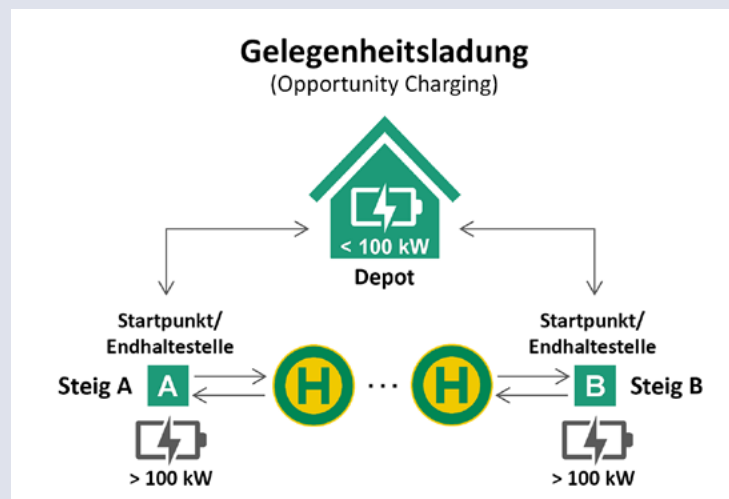
Abbildung 6: Schematische Darstellung des Ladekonzepts „Gelegenheitsladung“
