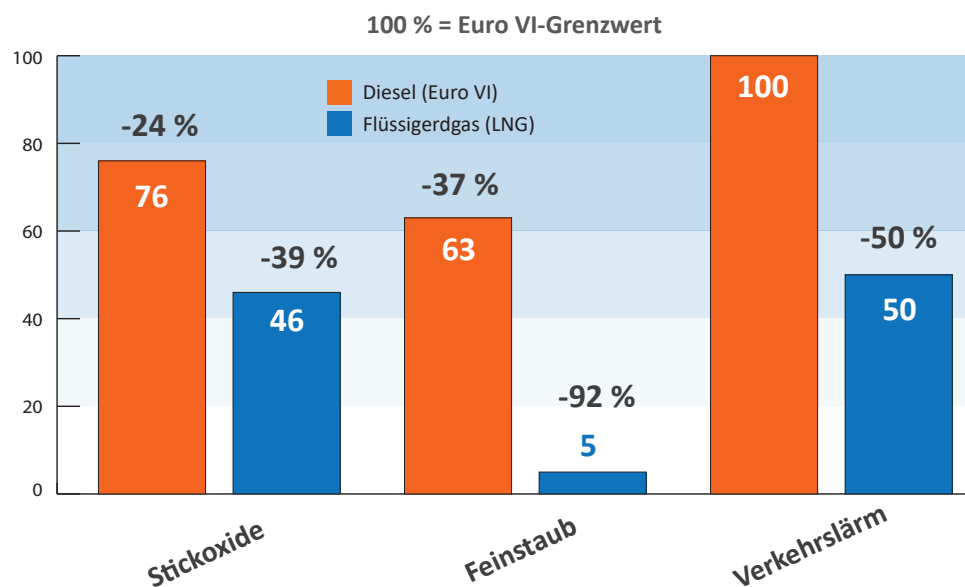
Abbildung 2: Emissionsvorteile von Gasantrieben gegenüber Euro VI-Dieselantrieben [9–11]
